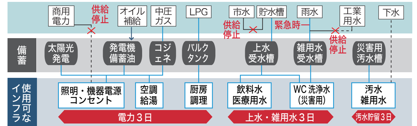
「災害自立運営型」病院の設備システム
